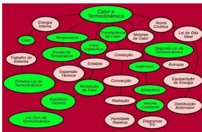
Figura 2. Mapa conceitual dos conteúdos da subárea Termodinâmica com base em Nave (2016) – tradução e adaptação dos autores.
